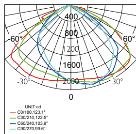
Curva fotométrica 50W
